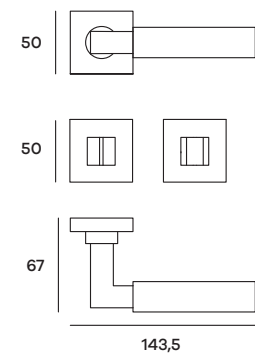
INFRO72W07 Maniglia su rosetta WC Doorhandle on WC rose
