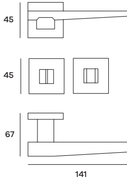
VETRO52W07 Maniglia su rosetta WC Doorhandle on WC rose
