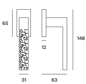
BILDK03 Maniglia per finestra DK Windowhandle DK
