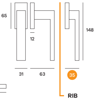
BILDK03 BILDK03-RIB Maniglia per finestra DK Windowhandle DK
