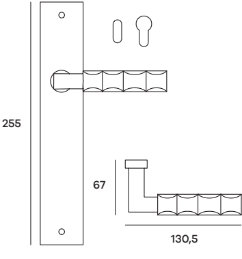
SNAPL51P (Patent) SNAPL51Y (Yale) Maniglia su placca Doorhandle on plate
