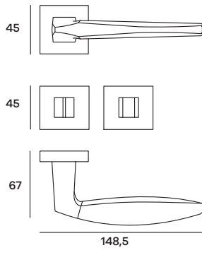
STORO52W07 Maniglia su rosetta WC Doorhandle on WC rose
