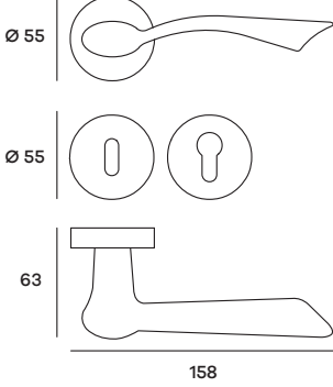
HELRO09P (Patent) HELRO09Y (Yale) Maniglia su rosetta Doorhandle on rose
