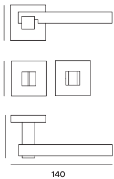
CODRO52W07 Maniglia su rosetta WC Doorhandle on WC rose
