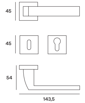
ZARRO57P (Patent) ZARRO57Y (Yale) Maniglia su rosetta Doorhandle on rose
