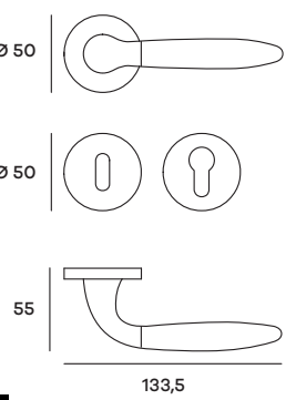
FUTRO04P (Patent) FUTRO04Y (Yale) Maniglia su rosetta Doorhandle on rose
