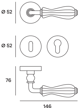
ZENRO97P (Patent) ZENRO97Y (Yale) Maniglia su rosetta Doorhandle on rose
