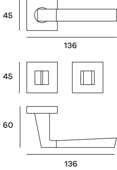
EASRO57W01 Maniglia su rosetta WC Doorhandle on WC rose
