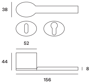
QUARO32P (Patent) QUARO32Y (Yale) Maniglia su rosetta Doorhandle on rose
