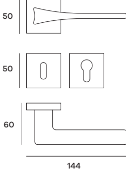
MALRO72P (Patent) MALRO72Y (Yale) Maniglia su rosetta Doorhandle on rose
