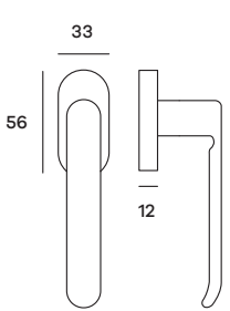
TEODK01 Maniglia per finestra DK Windowhandle DK
