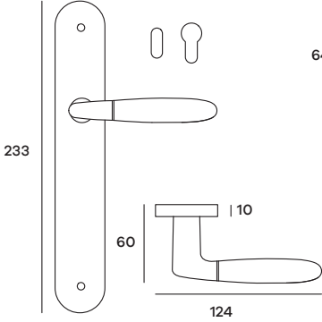
DR0PL15P (Patent) DR0PL15Y (Yale) Maniglia su placca Doorhandle on plate
