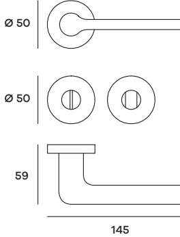
LINRO02W01 Maniglia su rosetta WC Doorhandle on WC rose
