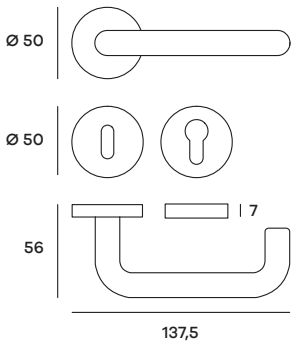
ATPRO02P (Patent) ATPRO02Y (Yale) Maniglia su rosetta Doorhandle on rose
