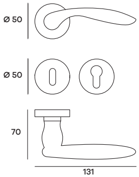
MIVRO06P (Patent) MIVRO06Y (Yale) Maniglia su rosetta Doorhandle on rose
