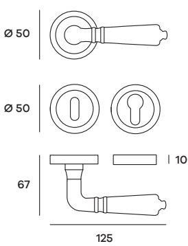
ANTRO07P (Patent) ANTRO07Y (Yale) Maniglia su rosetta Doorhandle on rose
