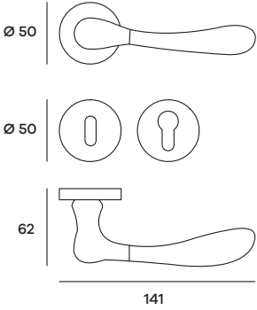
YARRO07P (Patent) YARRO07Y (Yale) Maniglia su rosetta Doorhandle on rose
