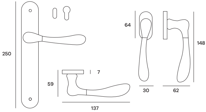
YARPL08P (Patent) YARPL08Y (Yale) Maniglia su placca Doorhandle on plate
