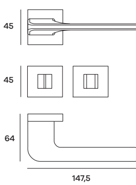
SIMRO52W07 Maniglia su rosetta WC Doorhandle on WC rose
