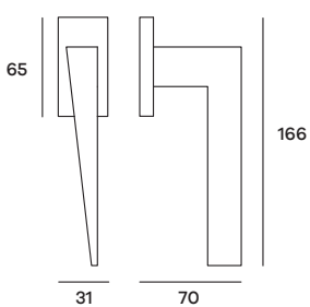
PHIDK03 Maniglia per finestra DK Windowhandle DK
