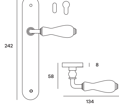
OTTPL02P (Patent) OTTPL02Y (Yale) Maniglia su placca Doorhandle on plate
