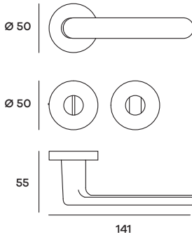
NEVRO02W01 Maniglia su rosetta WC Doorhandle on WC rose
