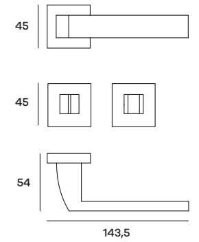
ZARRO57W07 Maniglia su rosetta WC Doorhandle on WC rose
