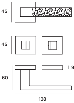
BILRO52W07 Maniglia su rosetta WC Doorhandle on WC rose
