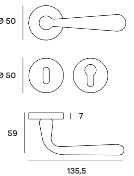
BRERO02P (Patent) BRERO02Y (Yale) Maniglia su rosetta Doorhandle on rose
