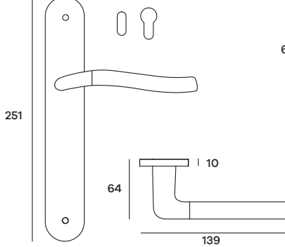
MOOPL05P (Patent) MOOPL05Y (Yale) Maniglia su placca Doorhandle on plate
