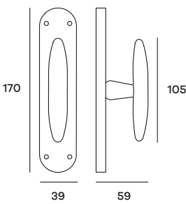
SABMRTCR02 Maniglia per cremonese Windowhandle
