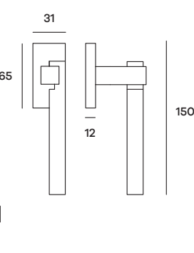
CODDK03 Maniglia per finestra DK Windowhandle DK
