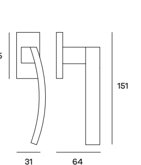
STYDK03 Maniglia per finestra DK Windowhandle DK
