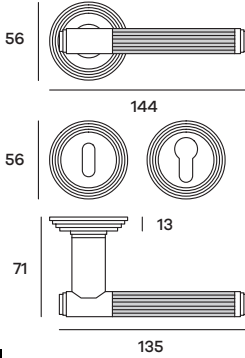
EXARO86P (Patent) EXARO86Y (Yale) Maniglia su rosetta Doorhandle on rose
