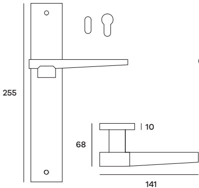
VETPL51P (Patent) VETPL51Y (Yale) Maniglia su placca Doorhandle on plate
