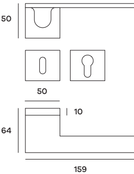
PLARO72P (Patent) PLARO72Y (Yale) Maniglia su rosetta Doorhandle on rose
