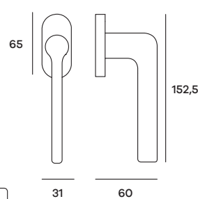
LINDK01 Maniglia per finestra DK Windowhandle DK
