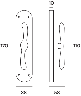
ASIMRTCR02 Maniglia per cremonese Windowhandle
