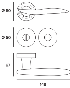
FLYRO15W01 Maniglia su rosetta WC Doorhandle on WC rose
