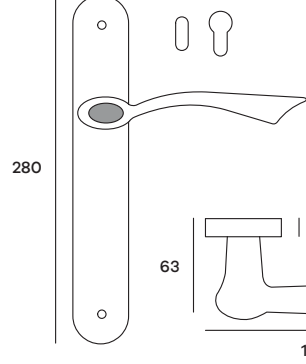
HELPL01P (Patent) HELPL01Y (Yale) Maniglia su placca Doorhandle on plate
