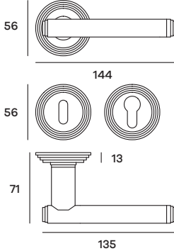
EXARO86P (Patent) EXARO86P (Yale) Maniglia su rosetta Doorhandle on rose
