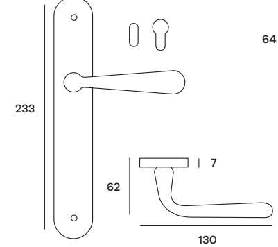
BREPL15P (Patent) BREPL15Y (Yale) Maniglia su placca Doorhandle on plate
