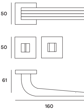
NAVRO52W07 Maniglia su rosetta WC Doorhandle on WC rose
