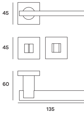
SQURO52W07 Maniglia su rosetta WC Doorhandle on WC rose
