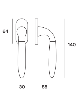
FUTDK01 Maniglia per finestra DK Windowhandle DK
