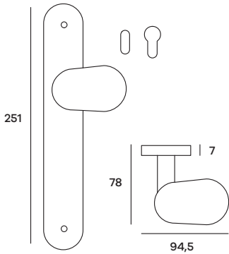
UOVPL05P (Patent) UOVPL05Y (Yale) Maniglia su placca Doorhandle on plate
