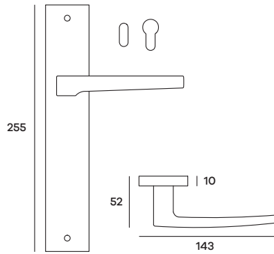
SYDPL51P (Patent) SYDPL51Y (Yale) Maniglia su placca Doorhandle on plate
