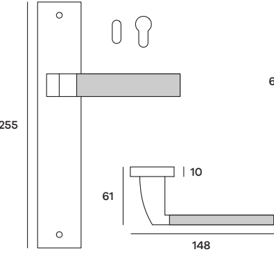
GENPL51P (Patent) GENRO51Y (Yale) Maniglia su placca Doorhandle on plate
