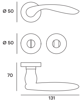
MIVRO06W01 Maniglia su rosetta WC Doorhandle on WC rose
