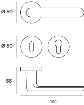
NEVRO02P (Patent) NEVRO02Y (Yale) Maniglia su rosetta Doorhandle on rose
