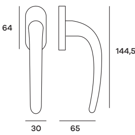
SABDK01 Maniglia per finestra DK Windowhandle DK
