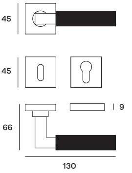
BOURO52P (Patent) BOURO52Y (Yale) Maniglia su rosetta Doorhandle on rose
