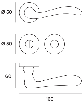
VERRO06W01 Maniglia su rosetta WC Doorhandle on WC rose
