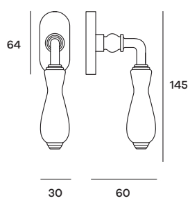
OTTDK01 Maniglia per finestra DK Windowhandle DK
