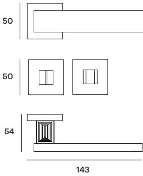
RMARO72W01 Maniglia su rosetta WC Doorhandle on WC rose
