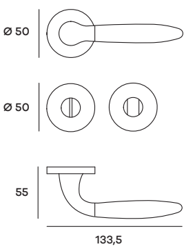
FUTRO04W01 Maniglia su rosetta WC Doorhandle on WC rose
