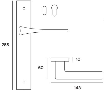
MALPL15P (Patent) MALPL15Y (Yale) Maniglia su placca Doorhandle on plate
