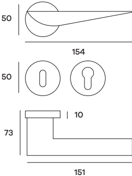
VEGRO03P (Patent) VEGRO03Y (Yale) Maniglia su rosetta Doorhandle on rose
