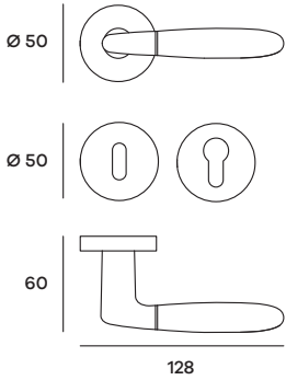
DRORO02P (Patent) DRORO02Y (Yale) Maniglia su rosetta Doorhandle on rose
