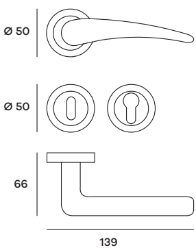
PHERO06P (Patent) PHERO06Y (Yale) Maniglia su rosetta Doorhandle on rose
