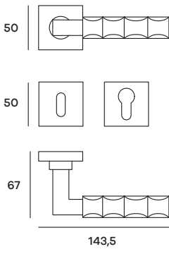
SNARO52P (Patent) SNARO52Y (Yale) Maniglia su rosetta Doorhandle on rose
