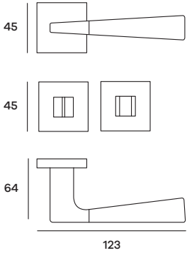
KUBRO52W07 Maniglia su rosetta WC Doorhandle on WC rose
