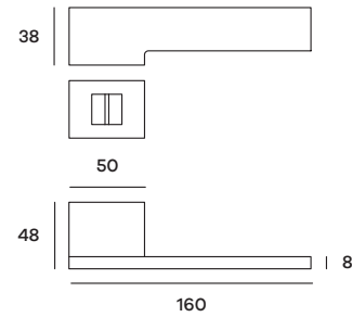
UNORO80W07 Maniglia su rosetta WC Doorhandle on WC rose
