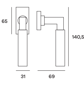
INFDK03 Maniglia per finestra DK Windowhandle DK
