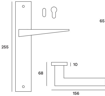
PHIPL51P (Patent) PHIPL51Y (Yale) Maniglia su placca Doorhandle on plate
