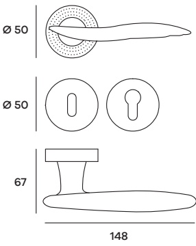
FLYRO15P (Patent) FLYRO15Y (Yale) Maniglia su rosetta Doorhandle on rose
