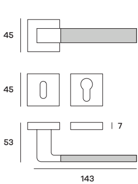
BIBRO57P (Patent) BIBRO57Y (Yale) Maniglia su rosetta Doorhandle on rose
