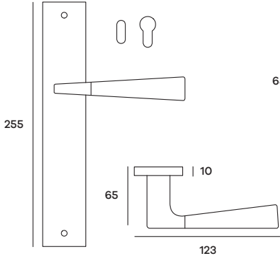
KUBPL15P (Patent) KUBPL15Y (Yale) Maniglia su placca Doorhandle on plate
