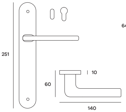
STIPL05P (Patent) STIPL05Y (Yale) Maniglia su placca Doorhandle on plate
