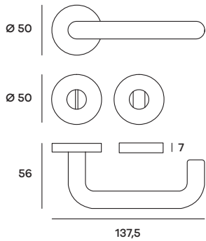
ATPRO02W01 Maniglia per WC Doorhandle WC
