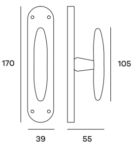
FUTMRTCR02 Maniglia per cremonese Windowhandle
