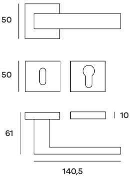
BILRO72P (Patent) BILRO72Y (Yale) Maniglia su rosetta Doorhandle on rose
