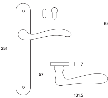
VERPL05P (Patent) VERPL05Y (Yale) Maniglia su placca Doorhandle on plate
