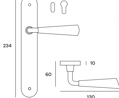
NILPL05P (Patent) NILPL05Y (Yale) Maniglia su placca Doorhandle on plate
