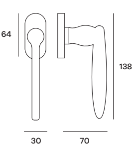
MIVDK01 Maniglia per finestra DK Windowhandle DK
