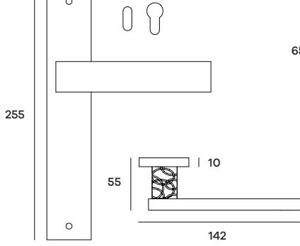
MUSPL52P (Patent) MUSPL52Y (Yale) Maniglia su placca Doorhandle on plate
