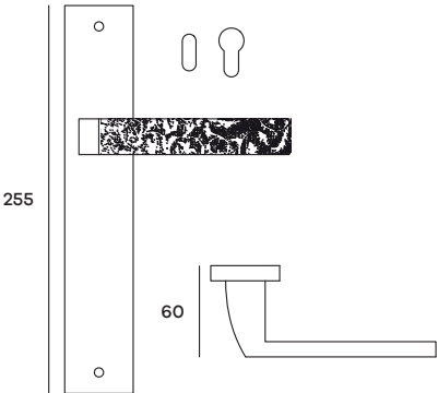
GENPL51P (Patent) GENRO51Y (Yale) Maniglia su placca Doorhandle on plate
