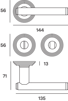
EXARO86W01 Maniglia su rosetta WC Doorhandle on WC rose
