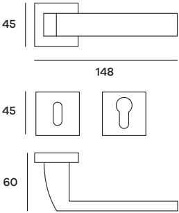
GENRO52P (Patent) GENRO52Y (Yale) Maniglia su rosetta Doorhandle on rose
