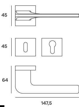
SIMRO52P (Patent) SIMRO52Y (Yale) Maniglia su rosetta Doorhandle on rose
