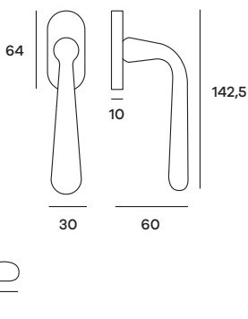
BREDK01 Maniglia per finestra DK Windowhandle DK
