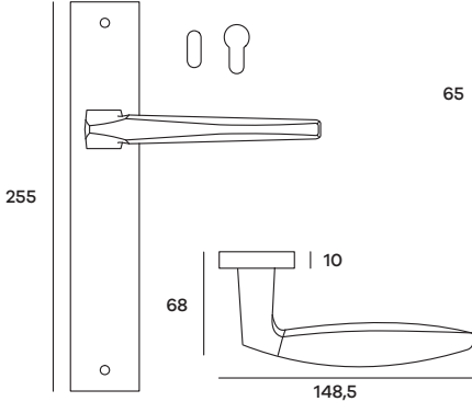
STOPL51P (Patent) STOPL51Y (Yale) Maniglia su placca Doorhandle on plate
