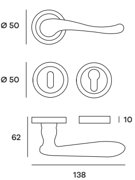
ASIRO07P (Patent) ASIRO07Y (Yale) Maniglia su rosetta Doorhandle on rose
