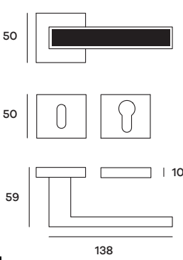
BILRO72P-A0 (Patent) BILRO72Y-A01 (Yale) Maniglia su rosetta Doorhandle on rose
