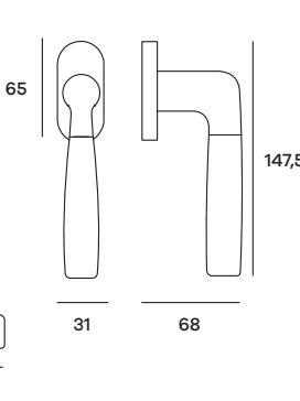
JETDK01 Maniglia per finestra DK Windowhandle DK
