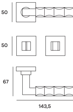
SNARO52W07 Maniglia su rosetta WC Doorhandle on WC rose
