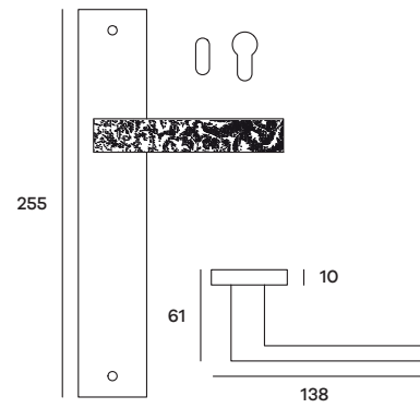
BILPL51P (Patent) BILPL51Y (Yale) Maniglia su placca Doorhandle on plate
