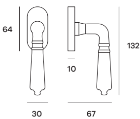
ANTDK01 Maniglia per finestra DK Windowhandle DK
