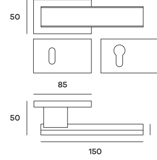
PENRO77P (Patent) PENRO77Y (Yale) Maniglia su rosetta Doorhandle on rose
