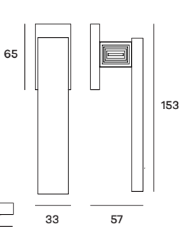
RMADK03 Maniglia per finestra DK Windowhandle DK
