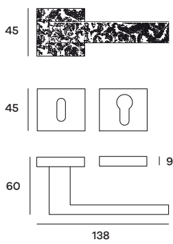
BILRO55W07 Maniglia su rosetta WC Doorhandle on WC rose
