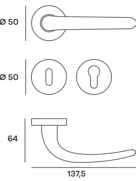
SABRO02P (Patent) SABRO02Y (Yale) Maniglia su rosetta Doorhandle on rose
