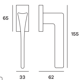
MALDK03 Maniglia per finestra DK Windowhandle DK
