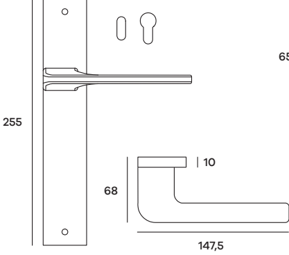
SIMPL51P (Patent) SIMPL51Y (Yale) Maniglia su placca Doorhandle on plate
