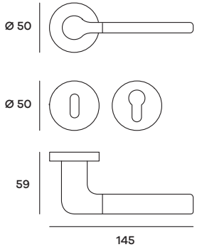
LINRO02P (Patent) LINRO02Y (Yale) Maniglia su rosetta Doorhandle on rose
