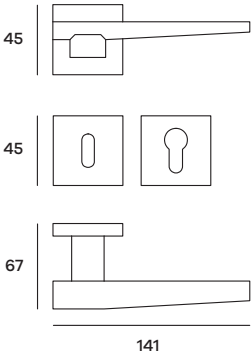
VETRO52P (Patent) VETRO52Y (Yale) Maniglia su rosetta Doorhandle on rose
