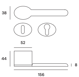
QUBRO32P (Patent) QUBRO32Y (Yale) Maniglia su rosetta Doorhandle on rose
