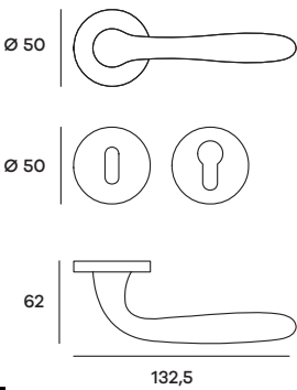
GOCRO02P (Patent) GOCRO02Y (Yale) Maniglia su rosetta Doorhandle on rose
