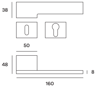
UNORO80P (Patent) UNORO80Y (Yale) Maniglia su rosetta Doorhandle on rose
