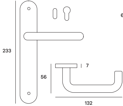
ATPPL15P (Patent) ATPPL15Y (Yale) Maniglia su placca Doorhandle on plate
