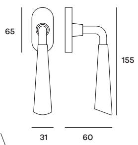
NILDK01 Maniglia per finestra DK Windowhandle DK
