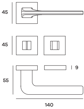
BOSRO52W07 Maniglia su rosetta WC Doorhandle on WC rose
