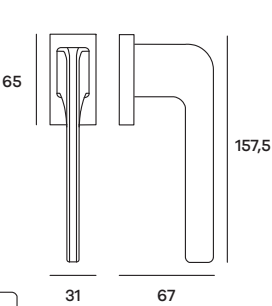
SIMDK03 Maniglia per finestra DK Windowhandle DK
