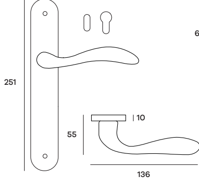
AURPL05P (Patent) AURPL05Y (Yale) Maniglia su placca Doorhandle on plate
