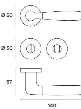
JETRO02W01 Maniglia su rosetta WC Doorhandle on WC rose
