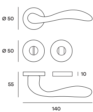
AURRO07W02 Maniglia per WC Doorhandle WC
