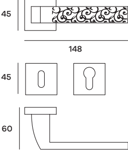
GENRO52P (Patent) GENRO52Y (Yale) Maniglia su rosetta Doorhandle on rose
