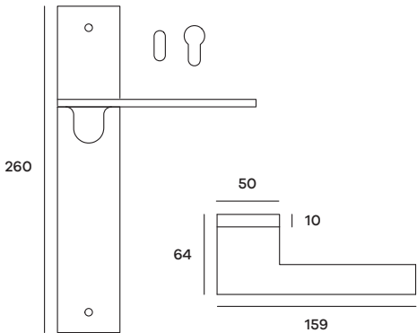
PLAPL59P (Patent) PLAPL59Y (Yale) maniglia su placca Doorhandle on plate
