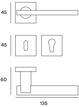
SQURO52P (Patent) SQURO52Y (Yale) Maniglia su rosetta Doorhandle on rose
