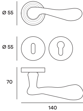
MAMRO15P (Patent) MAMRO15Y (Yale) Maniglia su rosetta Doorhandle on rose
