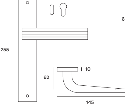
NAVPL51P (Patent) NAVPL51Y (Yale) Maniglia su placca Doorhandle on plate
