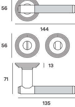
EXARO86W01 Maniglia su rosetta WC Doorhandle on WC rose
