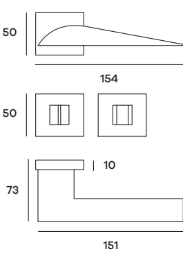
SAGRO72W07 Maniglia su rosetta WC Doorhandle on WC rose
