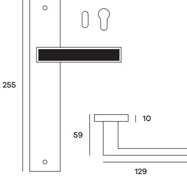
BILPL51-A01 (Patent) BILPL51Y-A01 (Yale) Maniglia su placca Doorhandle on plate
