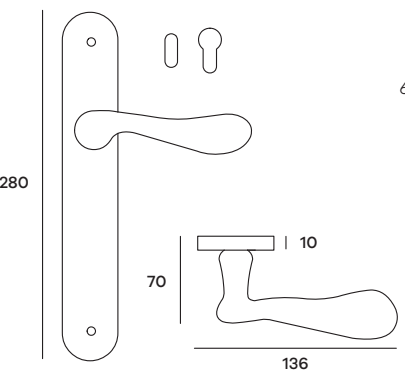
MAMPL01P (Patent) MAMPL01Y (Yale) Maniglia su placca Doorhandle on plate
