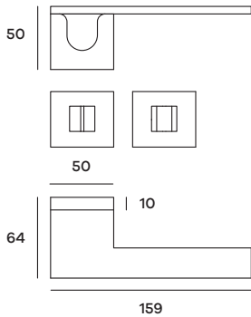
PLARO72W07 Maniglia su rosetta WC Doorhandle on WC rose
