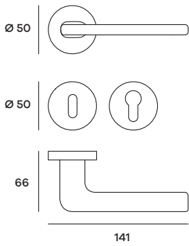
STIRO06P (Patent) STIRO06Y (Yale) Maniglia su rosetta Doorhandle on rose
