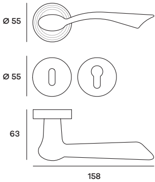
HELRO15P (Patent) HELRO15Y (Yale) Maniglia su rosetta Doorhandle on rose
