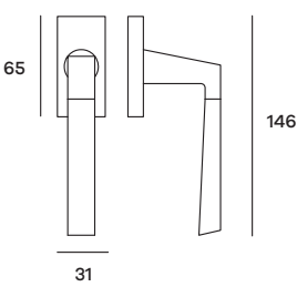
EASDK03 Maniglia per finestra DK Windowhandle DK
