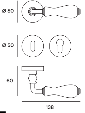
OTTRO07P (Patent) OTTRO07Y (Yale) Maniglia su rosetta Doorhandle on rose
