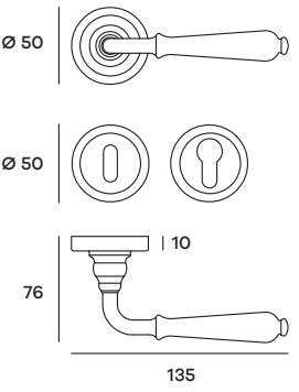
CLARO07P (Patent) CLARO07 (Yale) Maniglia su rosetta Doorhandle on rose
