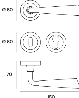
NILRO06P (Patent) NILRO06Y (Yale) Maniglia su rosetta Doorhandle on rose
