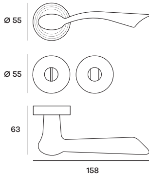
HELRO15W01 Maniglia su rosetta WC Doorhandle on WC rose
