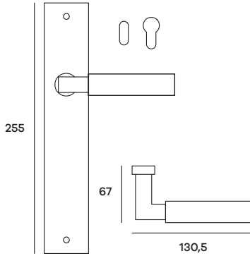
INFPL51P (Patent) INFPL51Y (Yale) Maniglia su placca Doorhandle on plate
