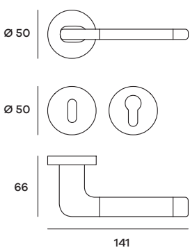
STIRO06P (Patent) STIRO06Y (Yale) Maniglia su rosetta Doorhandle on rose
