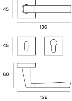
EASRO57P (Patent) EASRO57Y (Yale) Maniglia su rosetta Doorhandle on rose
