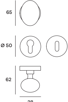
OVERO07P (Patent) OVERO07Y (Yale) Maniglia su rosetta Doorhandle on rose
