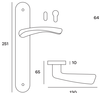
GALPL05P (Patent) GALPL05Y (Yale) Maniglia su placca Doorhandle on plate
