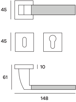
GENRO52P (Patent) GENRO52Y (Yale) Maniglia su rosetta Doorhandle on rose
