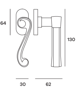
RICDK01 Maniglia per finestra DK Windowhandle DK
