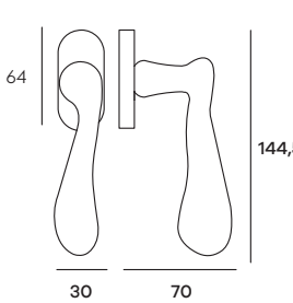
MAMDK01 Maniglia per finestra DK Windowhandle DK
