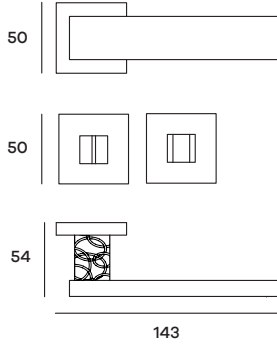
MUSRO72W01 Maniglia su rosetta WC Doorhandle on WC rose
