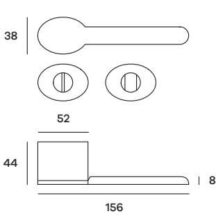
QUBRO32W01 Maniglia per WC Doorhandle WC
