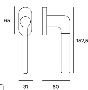
LINDK01 Maniglia per finestra DK Windowhandle DK
