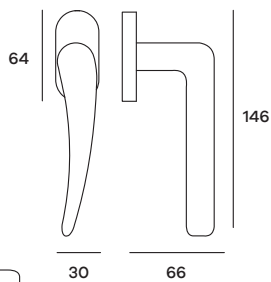
PHEDK01 Maniglia per finestra DK Windowhandle DK
