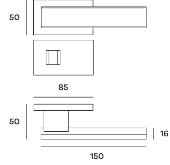
PENRO77W07 Maniglia su rosetta WC Doorhandle on WC rose
