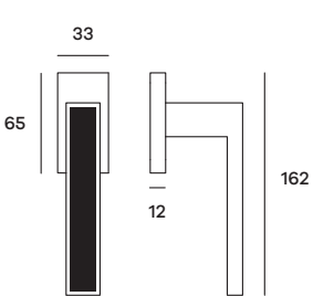
BILDK03-A01 Maniglia per finestra DK Windowhandle DK
