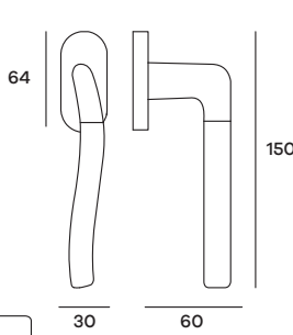
MOODK01 Maniglia per finestra DK Windowhandle DK
