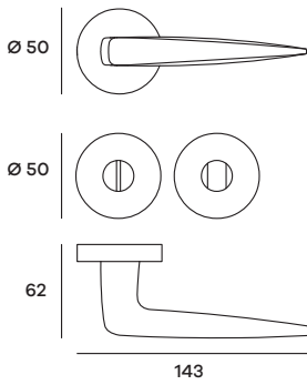
MIARO14W01 Maniglia su rosetta WC Doorhandle on WC rose
