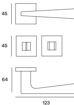
KUBRO52W07 Maniglia su rosetta WC Doorhandle on WC rose
