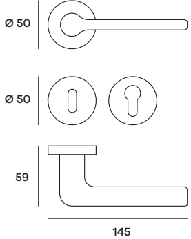
LINRO02P (Patent) LINRO02Y (Yale) Maniglia su rosetta Doorhandle on rose
