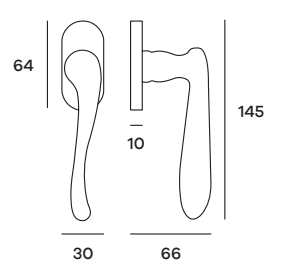
ASIDK01 Maniglia per finestra DK Windowhandle DK
