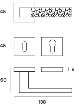
BILRO52P-A0 (Patent) BILRO52Y-A01 (Yale) Maniglia su rosetta Doorhandle on rose
