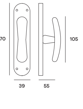
BREMTRC02 Maniglia per cremone Windowhandle
