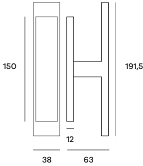
BILMRTC50 Maniglia per cremonese Windowhandle
