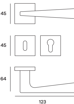
KUBRO52P (Patent) KUBRO52Y (Yale) Maniglia su rosetta Doorhandle on rose
