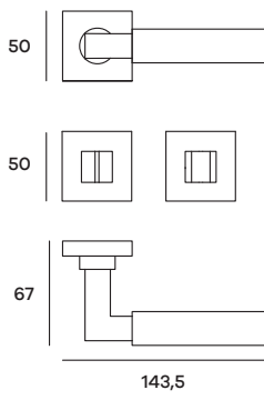
INFRO72W07 Maniglia su rosetta WC Doorhandle on WC rose
