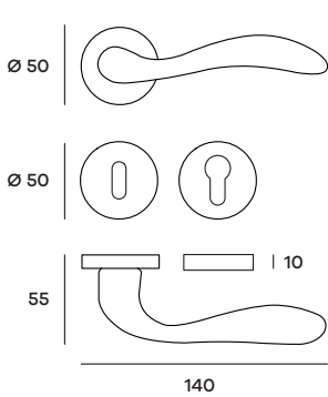
AURRO07P (Patent) AURRO07Y (Yale) Maniglia su rosetta Doorhandle on rose
