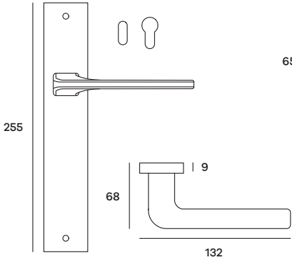
BOSPL51P (Patent) BOSPL51Y (Yale) Maniglia su placca Doorhandle on plate
