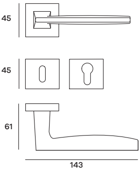
TECRO52P (Patent) TECRO52Y (Yale) Maniglia su rosetta Doorhandle on rose
