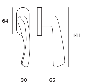
GALDK01 Maniglia per finestra DK Windowhandle DK
